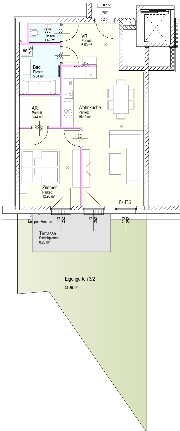
ÜBERSICHTSPLAN (Maßstabslos)
